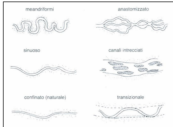
Figura 10 - Tipi morfologici
